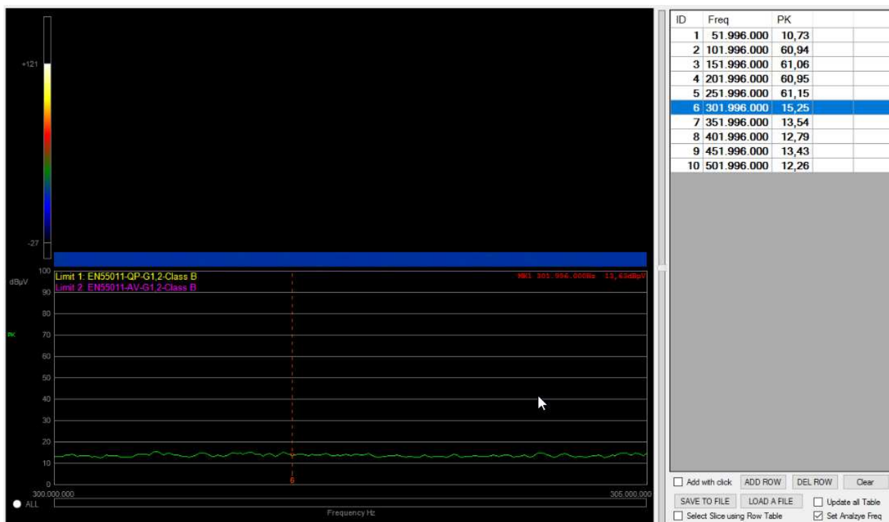
Fig. D.82: Set Analyze Freq
